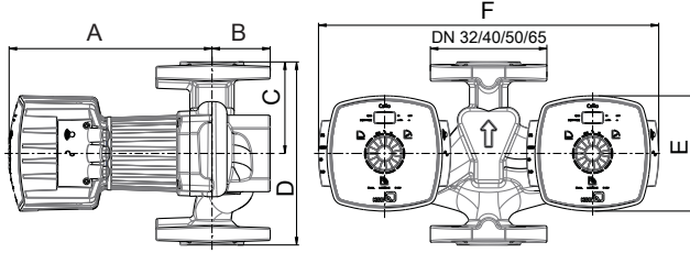
Şek. 5: Flanş bağlantısına sahip pompa agregası
