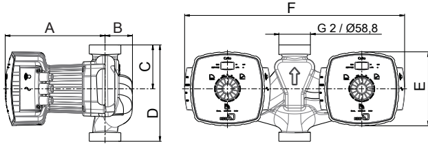
Şek. 4: Dişli bağlantısına sahip pompa agregası
