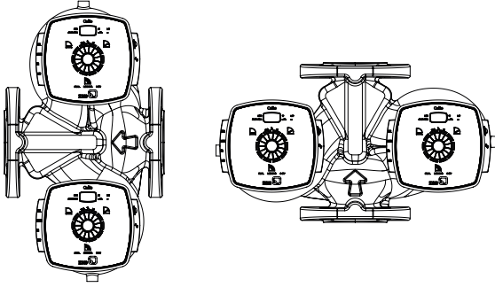
Şek. 6: İzin verilen montaj konumları
